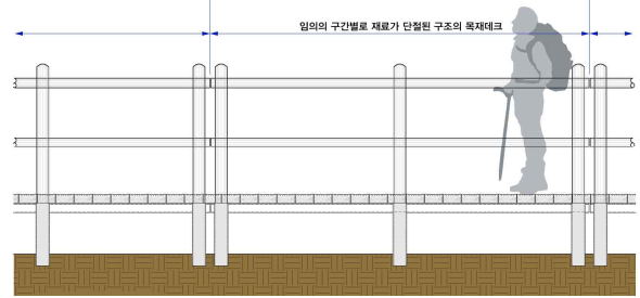
▲ (개선) 임의의 구간별로 모듈을 정하여 재료가 단절된 구조의 목재데크
